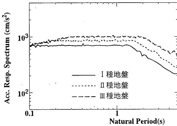
図-4.8-a 加速度応答スペクトル
