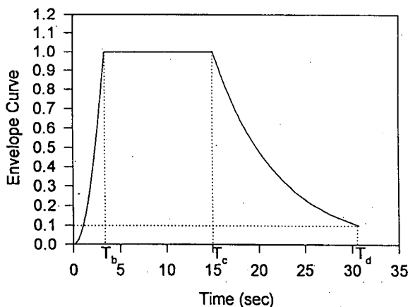
(a) 包絡線関数
