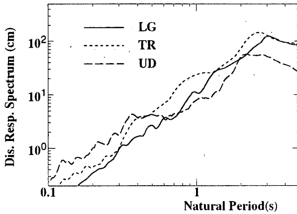
図-4.6-c 変位応答スペクトル
