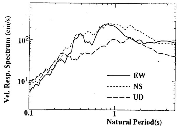
図-4.5-b 速度応答スペクトル
