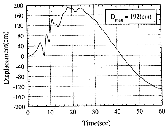
(a) 時間領域での積分：基準線補正
