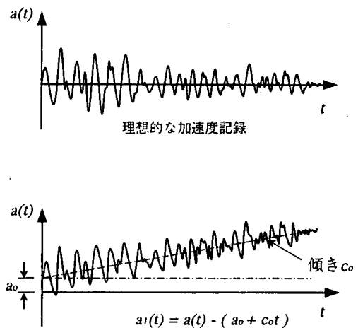
図4-10 加速度波形の基準線補正
