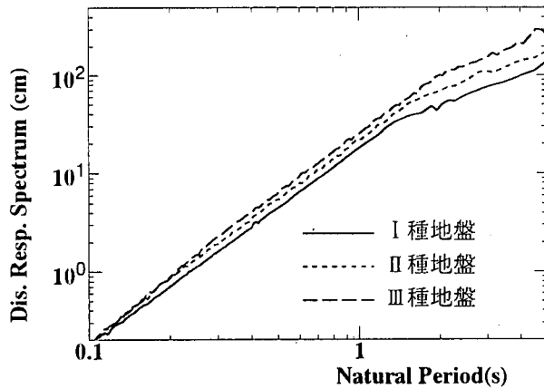
図-4.8-c 変位応答スペクトル
