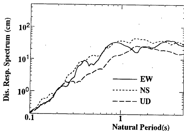
図-4.5-c 変位応答スペクトル
