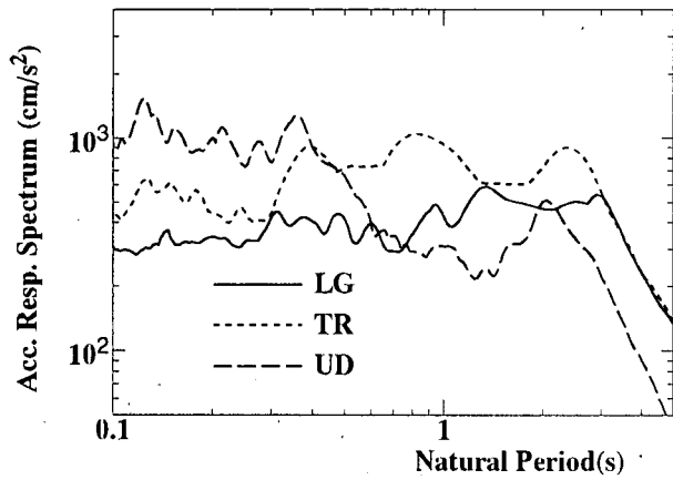
図-4.6-a 加速度応答スペクトル
