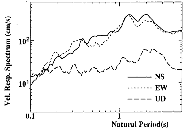
図-4.7-b 速度応答スペクトル
