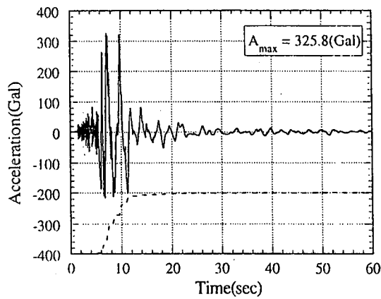
図4-12 加速度波形の一例
