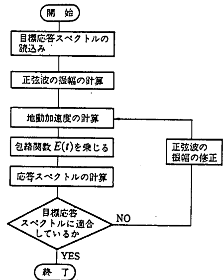
図4-16 正弦波合成法による模擬波形発生手順
