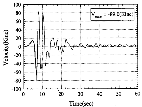
(b) 周波数領域での積分
