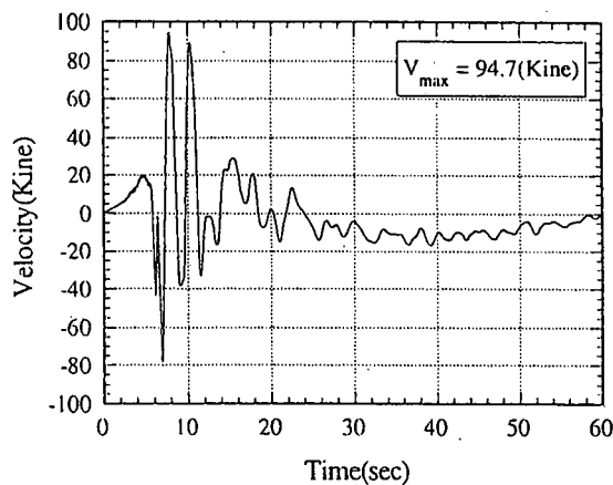
(a) 時間領域での積分
