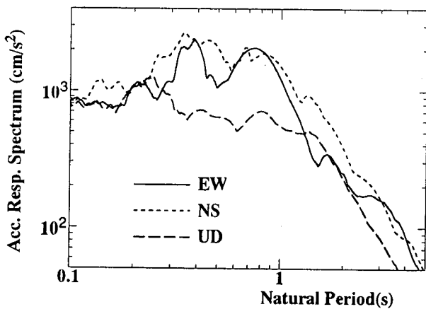
図-4.5-a 加速度応答スペクトル
