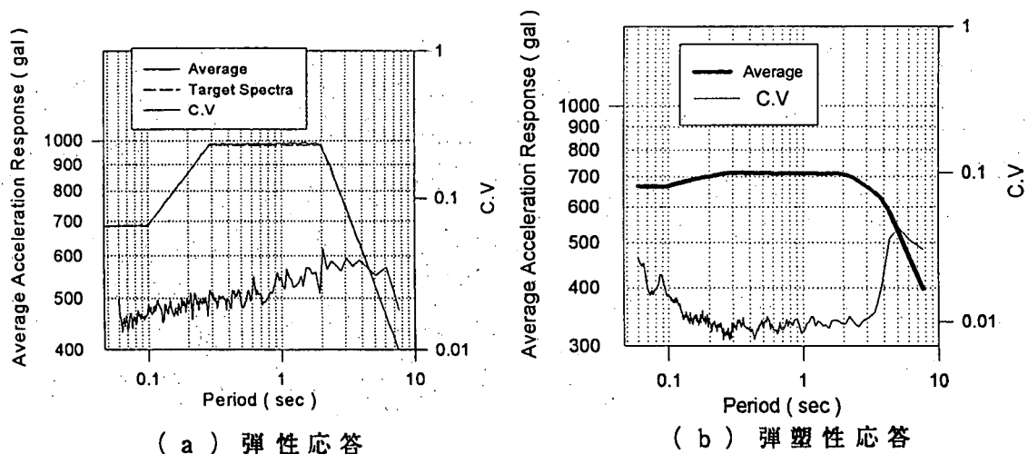
図 4 - 2 0 加速度応答の平均値と変動係数
