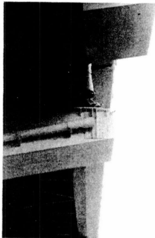
写真6-1 支承の損傷
