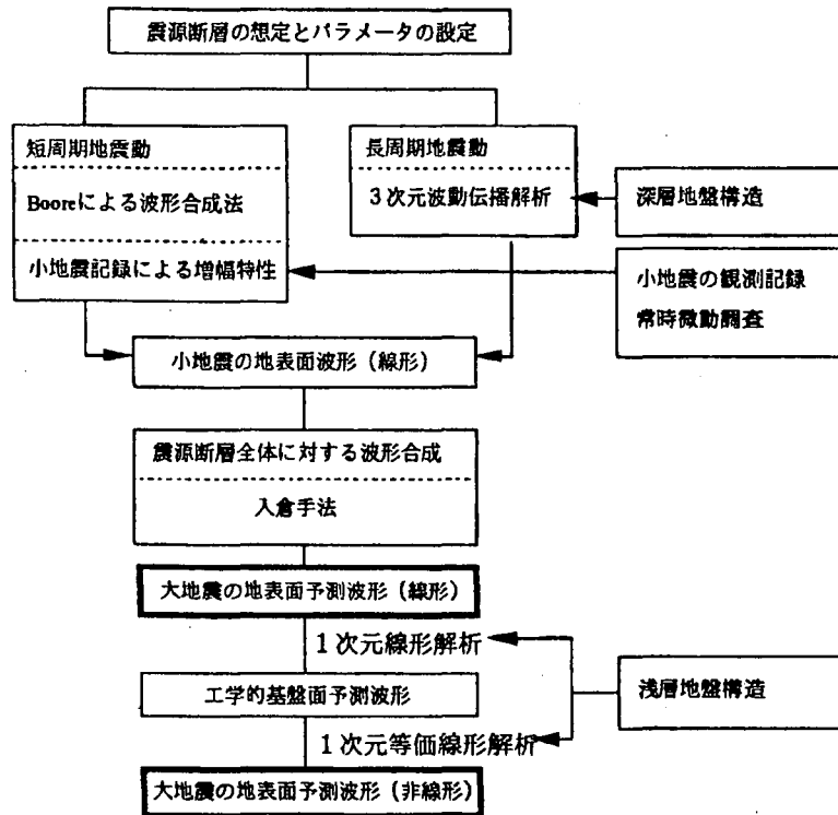
図-3.5.7 大阪府土木部の地震動計算フロー 20)
