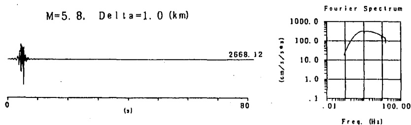
図-3.4.7 \omega^{-2} 則を満たす加速度波形
