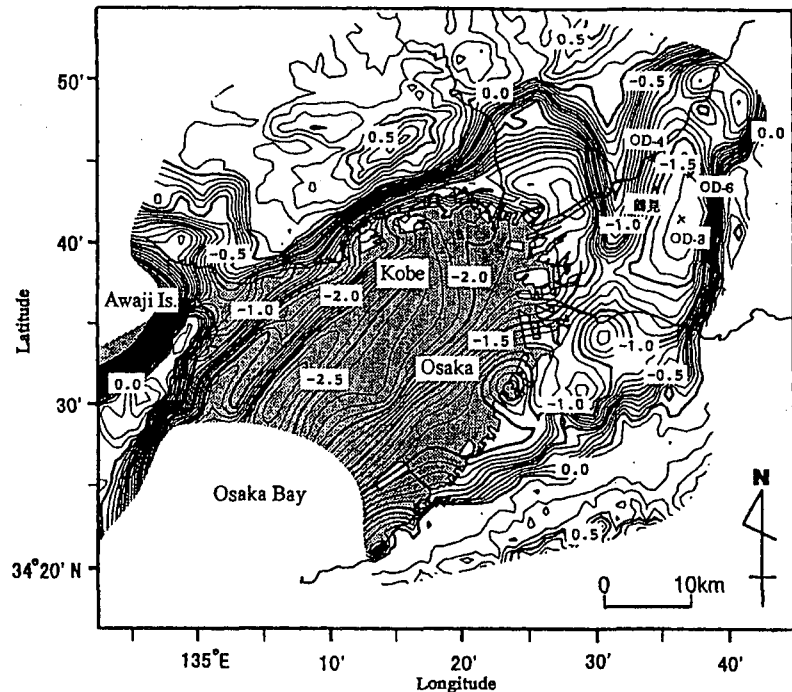
図-3.5.2 重力異常による大阪地域の基盤岩深度構造 15)
