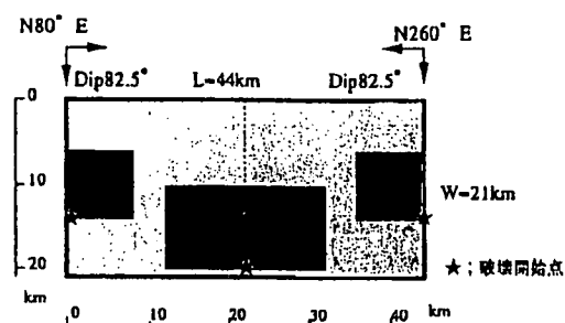
図-3.5.9 非一様すべり分布例 20)
