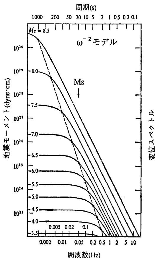
図-3.4.4 震源から放射される地震波のフーリエ変位スペクトル
