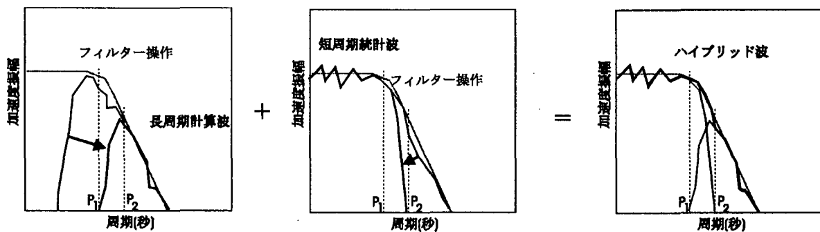
図-3.4.8 ハイブリッド法による長周期波と短周期波の足し合わせ
