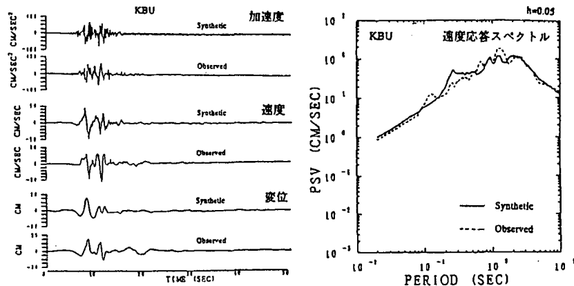
図-3.5.1 平成7年兵庫県南部地震の強震動シミュレーション例 11)
