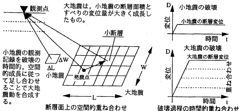
図-3.4.3 経験的グリーン関数合成法の内容
