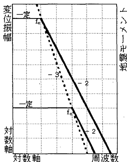
図-3.4.5 変位スペクトルの相似則
