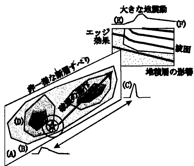
図-3.3.8 平成7年兵庫県南部地震による強震動の生成
