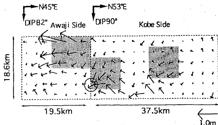
図-3.3.6 平成7年兵庫県南部地震で推定されている断層すべり分布 2)
