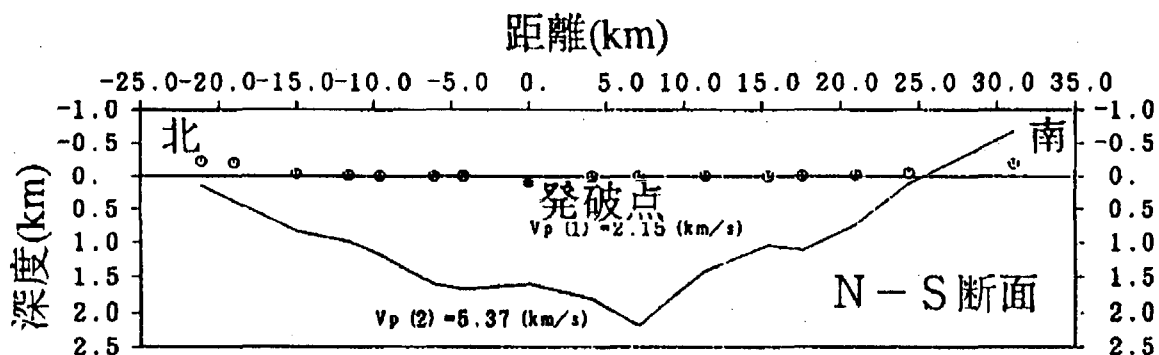
図-3.5.3 屈折法地震探査で推定した大阪平野の基盤岩深度南北断面 16)
