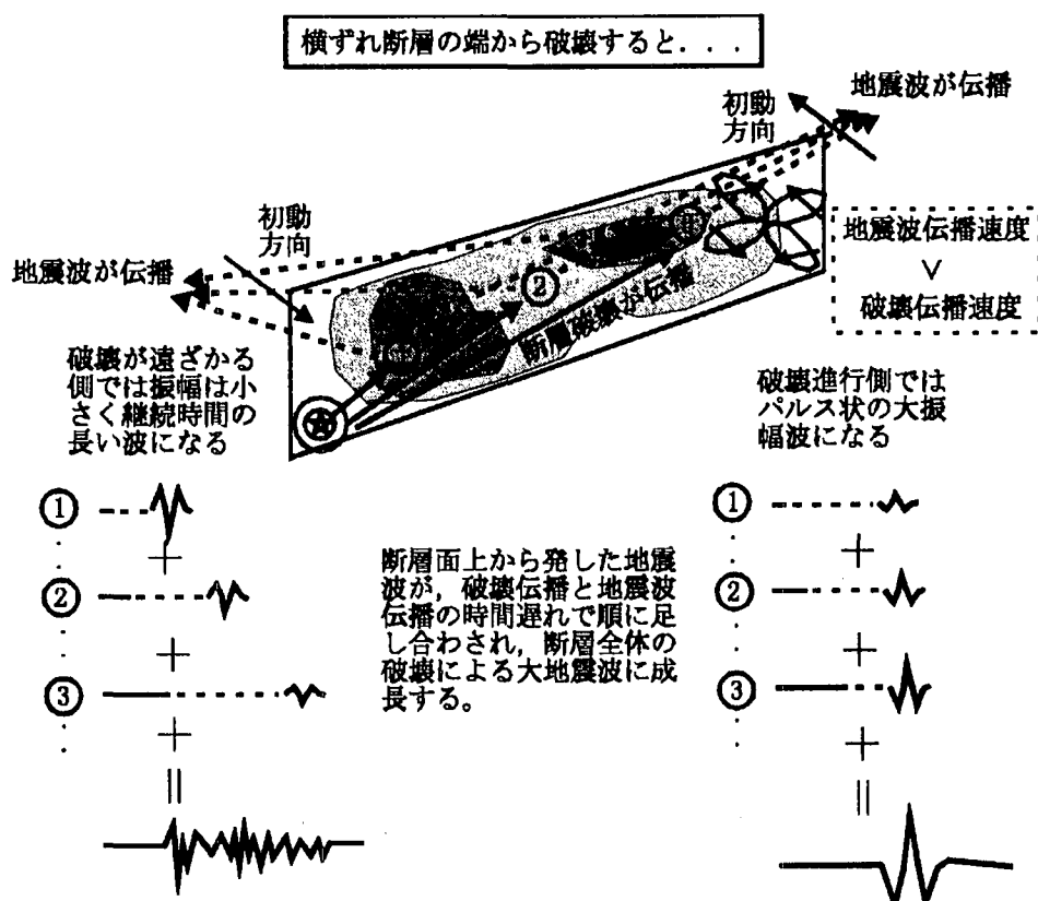
図-3.3.4 断層面上の破壊の進行と観測される地震波の特徴（断層端から）
