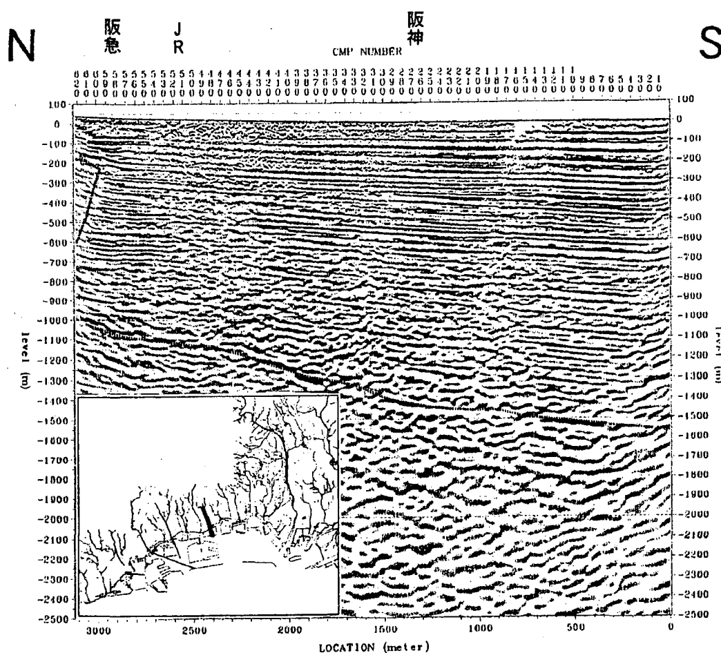
図-3.5.4 反射法地震探査による神戸地域の深層地盤構造 17)
