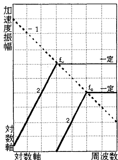
図-3.4.6 加速度スペクトルの相似則
