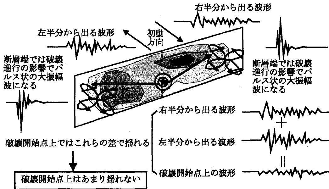
図-3.3.5 断層面上の破壊の進行と観測される地震波の特徴（断層中央から）
