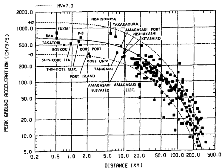
図-3.4.1 平成 7 年兵庫県南部地震による最大加速度の距離減衰 5)
