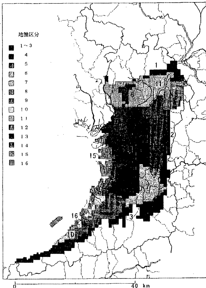
図-3.5.10 大阪府土木部のゾーン分割 20)
