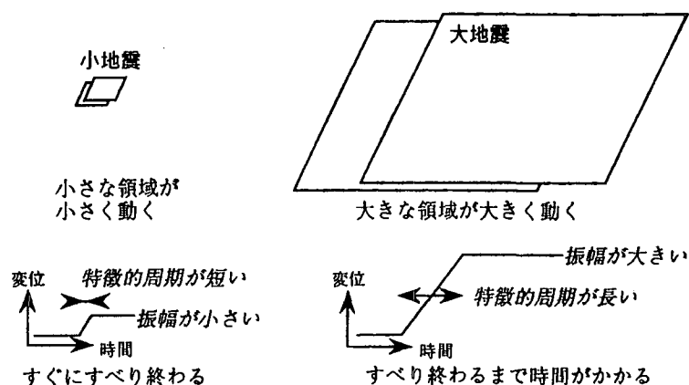
図-3.4.2 小地震と大地震の違い
