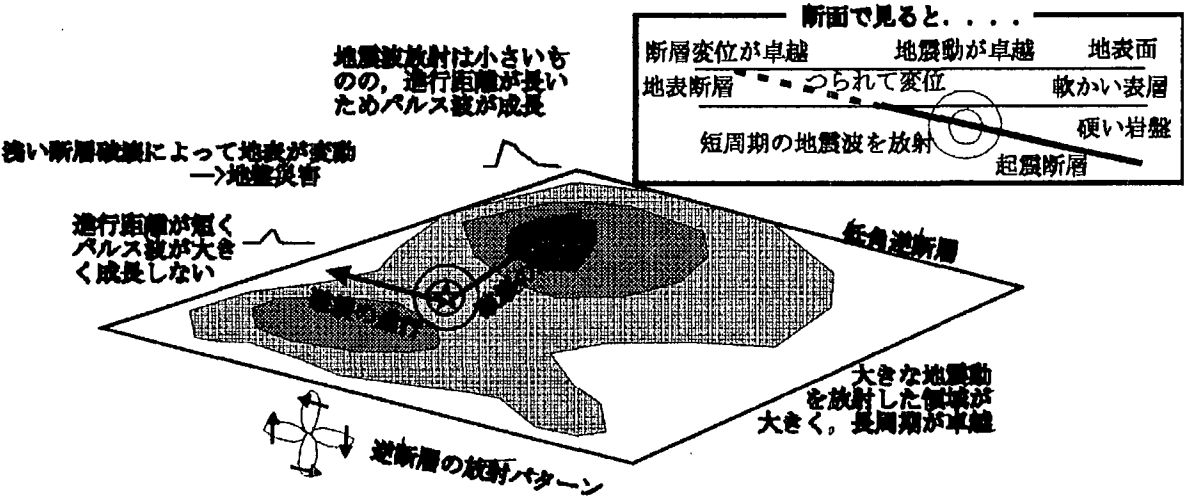
図-3.3.9 1999 年台湾集集地震による強震動の生成
