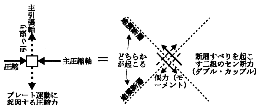
図-3.3.2 力の方向と断層の破壊面
