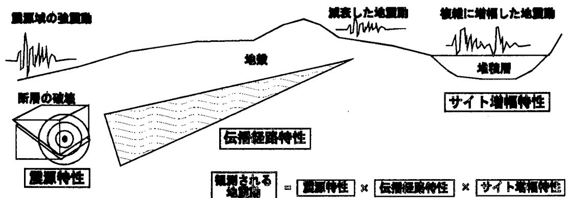
図-3.2.1 地震現象の概念（左：震源特性，中：伝播経路特性，右：地盤増幅特性）
