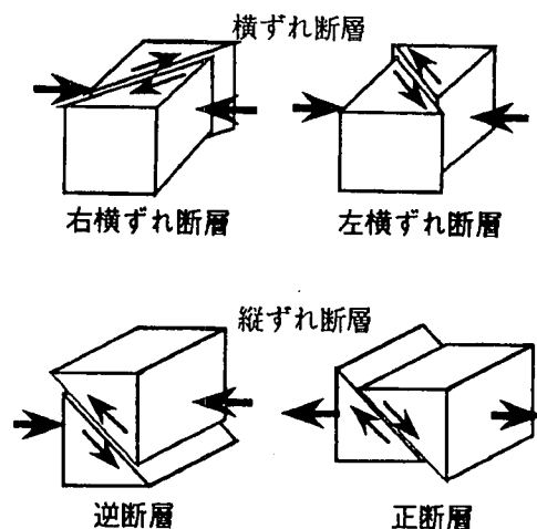
図-3.3.1 地震断層の種類
