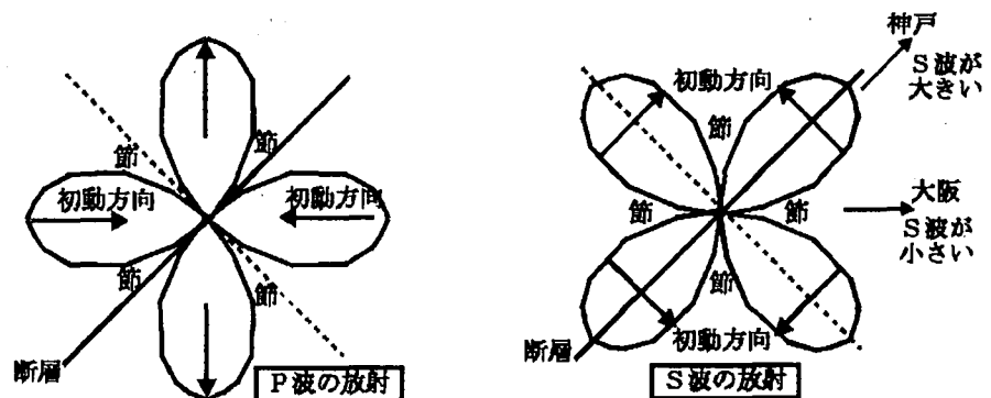
図-3.3.3 断層から放射される地震波
