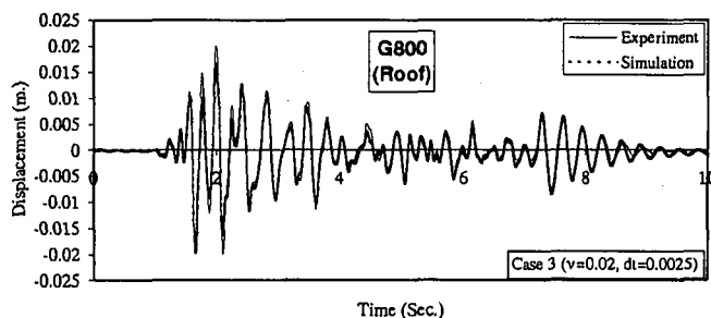
図-23 振幅800Galにおける変位応答(屋上) (減衰2%, 時間増分=0.0025s)
