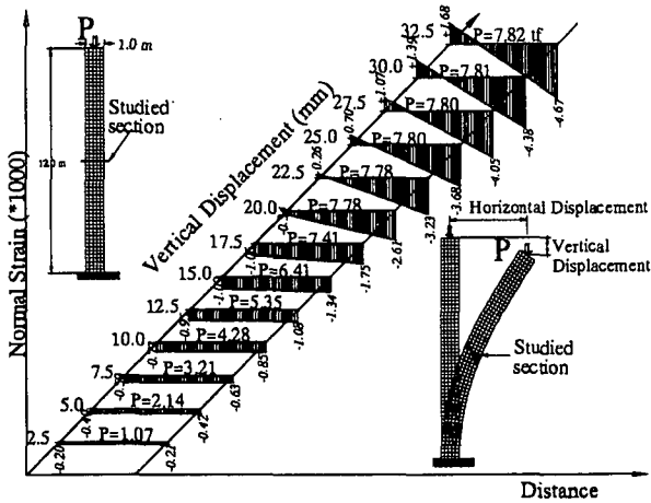
図-15 载荷荷重の増加に伴って生じる偏心荷重
