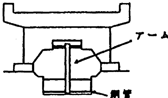
図-5.2.12 吸震装置
