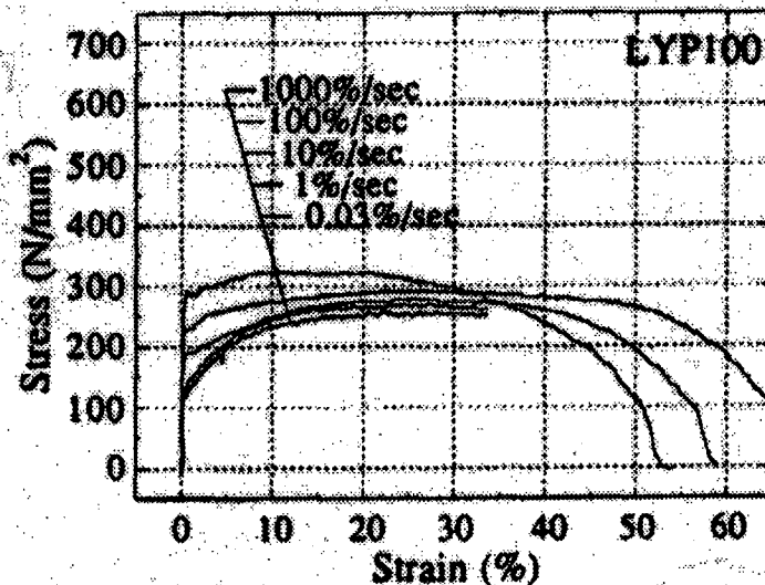
図-5.1.6 歪み速度の降伏強度に与える影響
