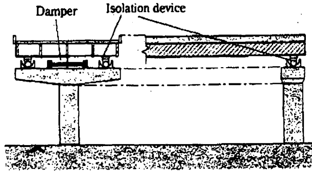
図-5.2.11 免震装置
