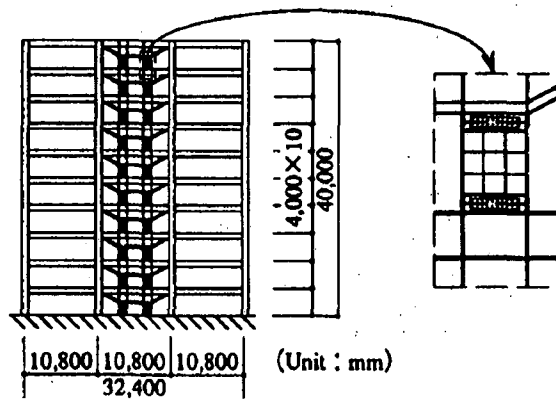
図-5.2.2 鋼板パネル付き建築骨組
