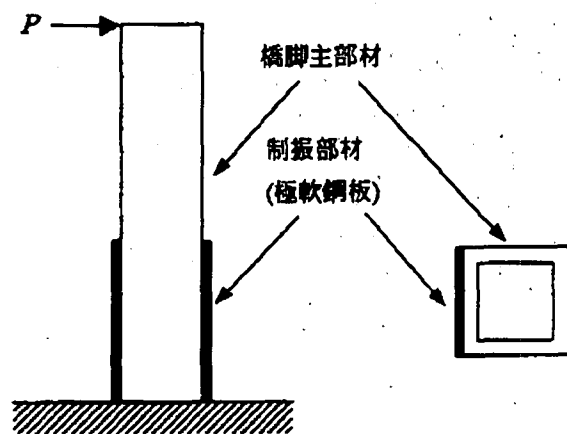
図-5.2.9 制震部材
