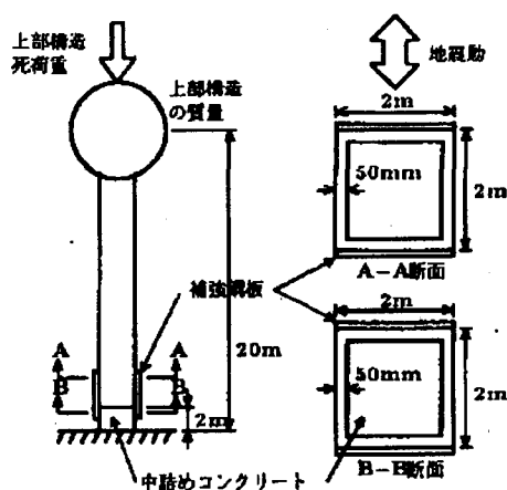
図-5.2.10 補強部材
