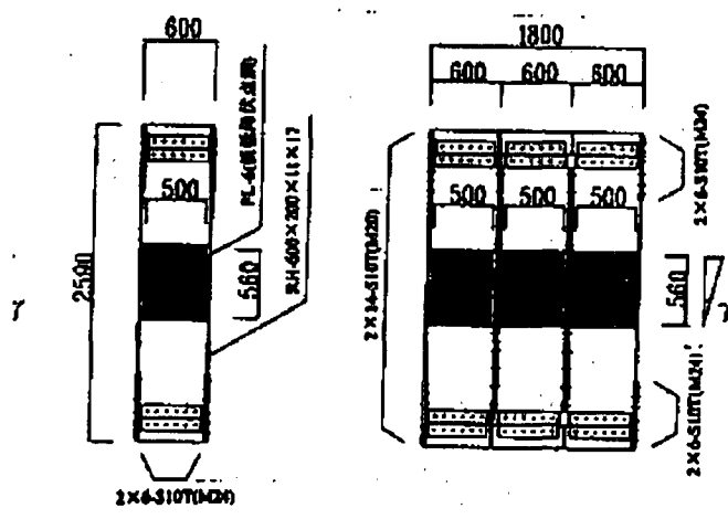
図-5.2.4 制震壁
