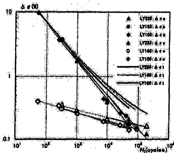
図-5.1.5 Manson-coffin 則による疲労寿命評価
