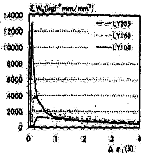
図-5.1.4 エネルギー吸収能力
