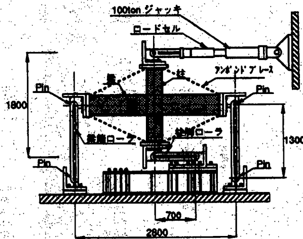
図4 加力装置
