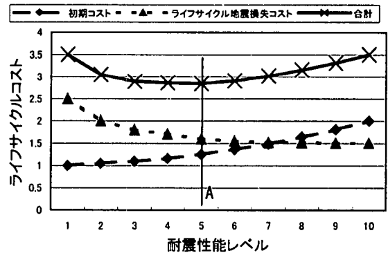
図-12 最適耐震性能の検討図
