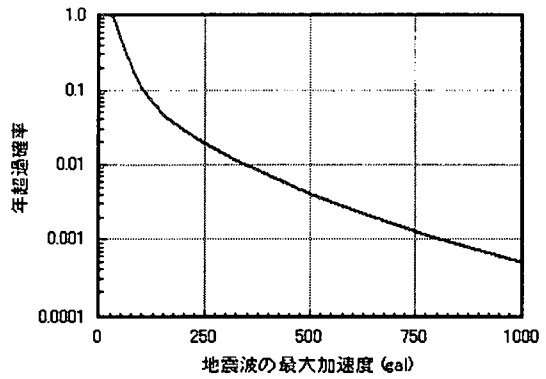
【ハザード曲線】
