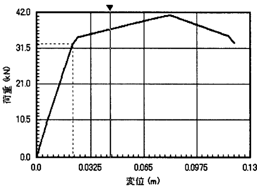
【荷重-変位】
