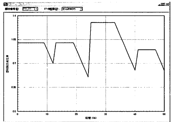
図-8 構造物の耐力低下/回復の設定例
