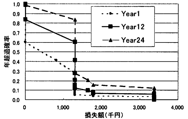
図-11 リスクカーブ (Year1, 12, 24)
