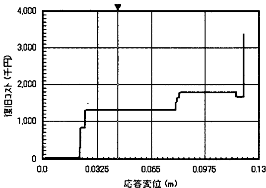
【復旧コスト-応答変位】
