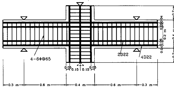
図-9 RC 構造の柱-梁接合部の交番载荷実験の供試体
