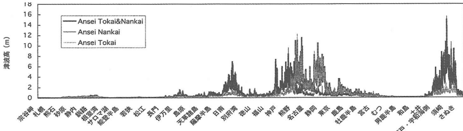
図-4 1854年安政モデルの同時発生時と東海地震・南海地震単独発生時の津波高の比較
