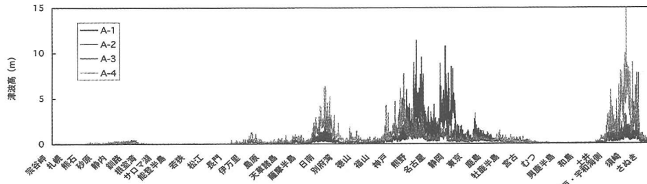
図-5 各セグメントのみで地震が発生した場合の津波高 (1854年安政モデル)
