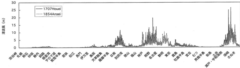
図-3 1707年宝永モデルと1854年安政モデルの同時発生時の津波高の比較
