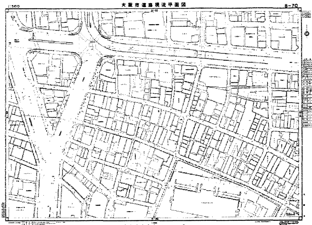
図 7: 大阪市土木技術協会 [15] 提供の道路現況平面図 (同 web site[15] より引用)
