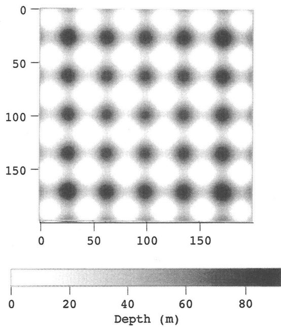
図 9: 島を含む仮想地形
