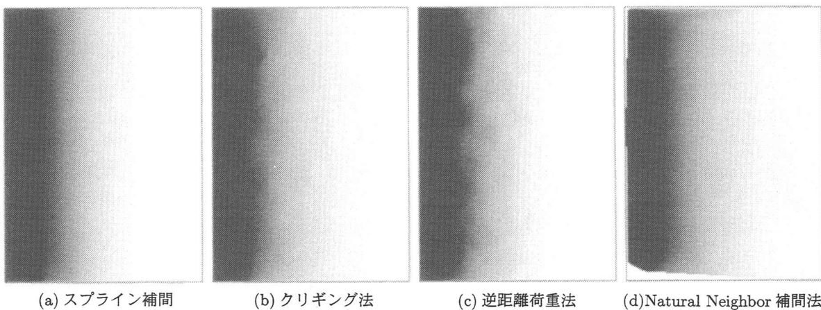
図 10: 陸を含む仮想地形の再現性
