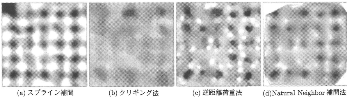
図 11: 島を含む仮想地形の再現性
