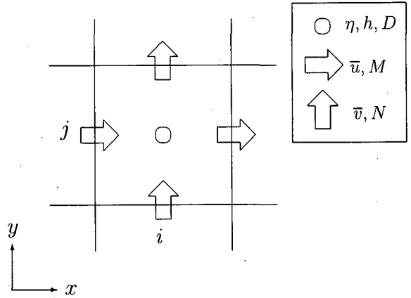
図 2: スタガード格子における変数の配置
