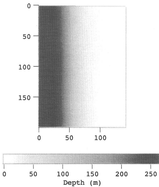
図 8: 陸を含む仮想地形
