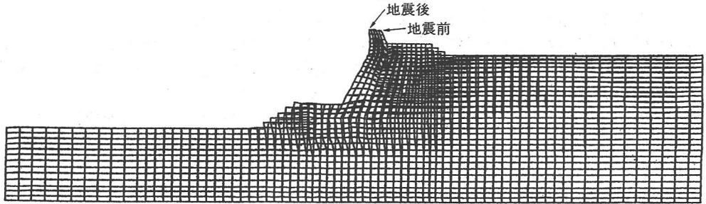
(a) 現地地盤での条件の解析結果
