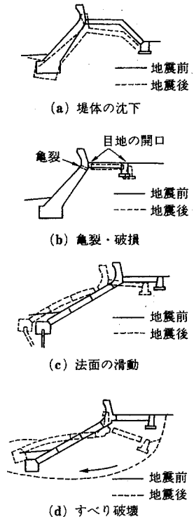
図-1 土堰堤式構造物の変形形態
