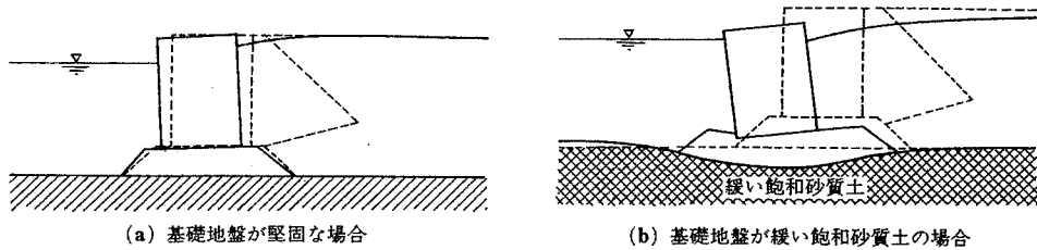
図-2 重力構造物の変形形態
