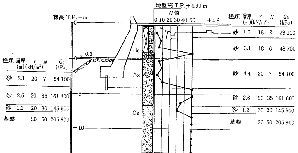
図-7 耐震性能照査の対象断面
