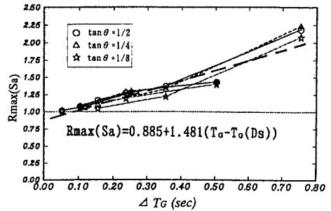
図-2 R_{max}(Sa) と \Delta T_G の関係
