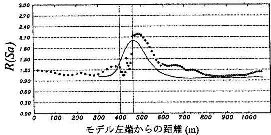
図-4 R(Sa) の分布(推定値と計算値の比較)
