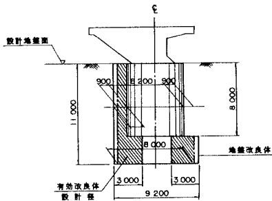
図-4 地盤改良の概要
