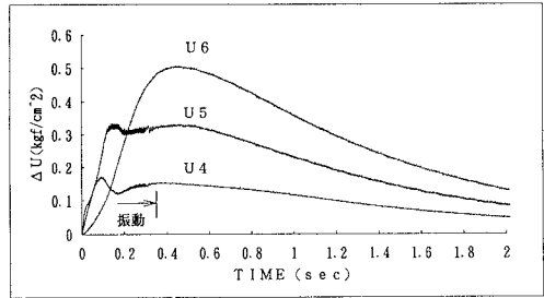
図-2 間隙水圧の経時変化
