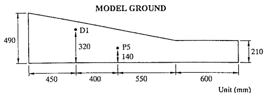
図1: 模型地盤
