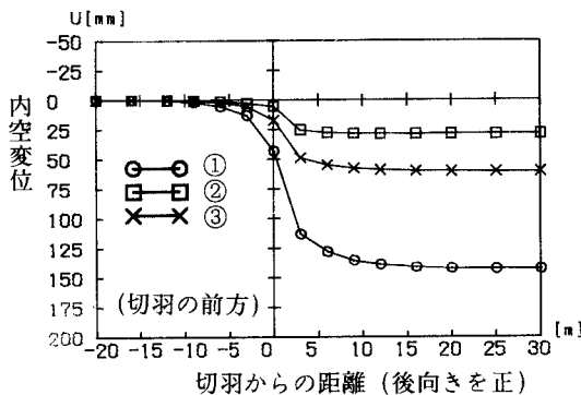
図-5 内空変位分布（解析1：無支保）
