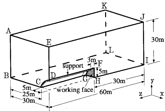
図-1 解析領域
