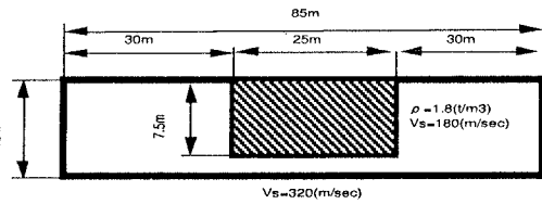
図-6 解析断面
