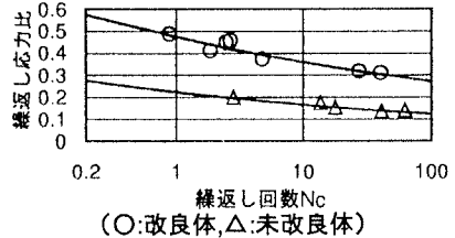
図-2 液状化強度曲線
