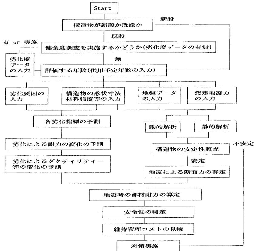
図-1 コンクリート構造物の健全度考慮した耐震評価のフロー
