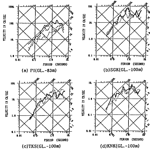
図-2 最深部(GL-100m)の疑似速度応答スペクトル(h=7%) (実線:NS,一点鎖線:EW,点線:UD)
