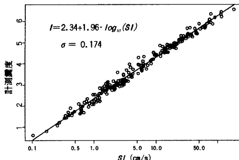
図4 SI値と計測震度
