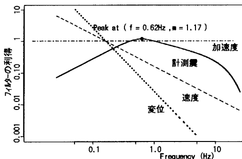
図1 計測震度のフィルタと速度、加速度フィルタの比較
