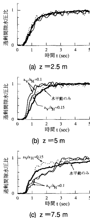
図-5 傾斜加振時の過剰間隙水圧比の推移 ( a_{Hmax} = 0.12G )
