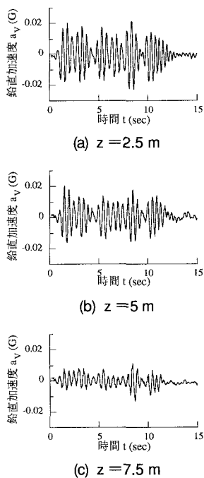
図-4 傾斜加振時の鉛直加速度の伝播
