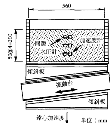
図-3 遠心力場における傾斜加振実験の方法および供試体の概観
