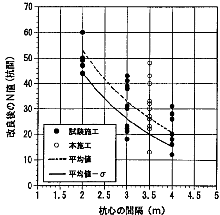
図-6 鋼管杭打設間隔と杭間のN値
