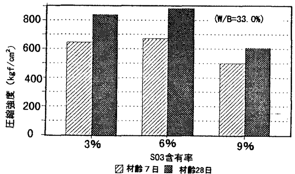
図-4 自己充填型高流動コンクリートのSO 3 含有率と圧縮強度の関係
