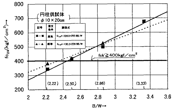
図-3 圧縮強度とW/Bとの関係
