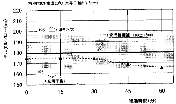
図-2 軽量繊維補強モルタルのフロー値の経時変化
