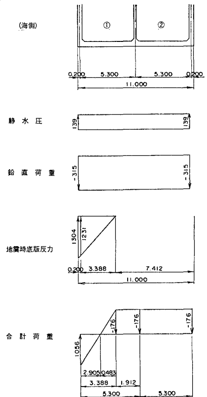
図-1 底版作用荷重(kN/m 2 )
