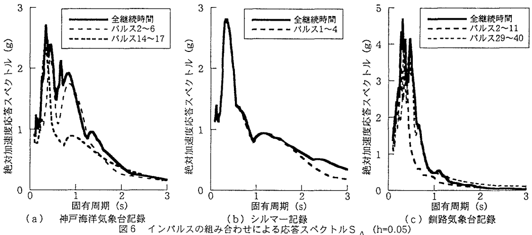
図6 インパルスの組み合わせによる応答スペクトル S_A ( h=0.05 )
