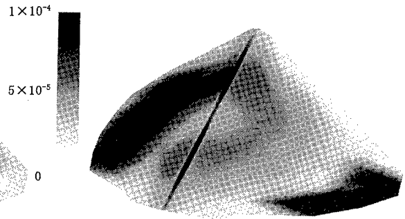
図3 最大ひずみ分布
