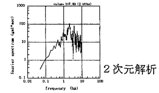
図5 天端中央部における加速度フーリエスペクトル
