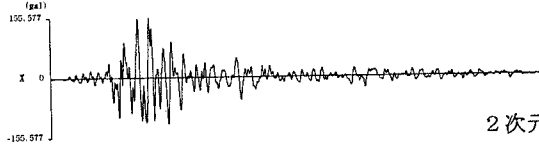
図4 天端中央部における加速度波形
