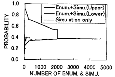
図2 状態列挙とモンテカルロ法によるシステム信頼度 ( p = 0.9, r = 80\% )
