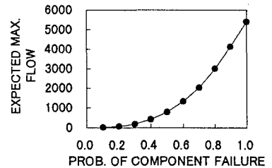
図4 リンク信頼度と期待最大フロー
