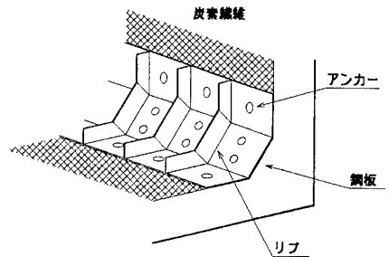
図-6 リブ付き鋼板
