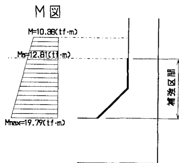
図-3 補強範囲
