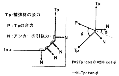
図-4 アンカーの引抜き
