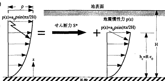
図-2 解析で考慮すべき集中せん断力と分布地震慣性力
