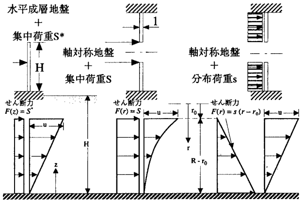
図-3 集中せん断力 S^* の変換
