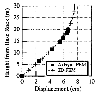
図-5 地盤変位の鉛直分布
