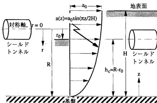
図-1 軸対称モデルの概念図
