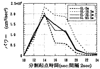
図-4 分割パワーの時間推移
