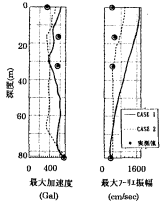
図-3 深度~最大加速度、最大フーリエ振幅関係(CASE1,2)
