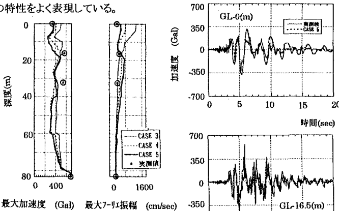
図-5 深度~最大加速度、最大フーリエ振幅関係(CASE3,4,5)
