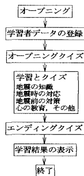
図1 ソフトウェアの流れ
