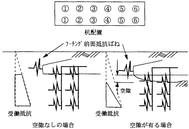
図5. 空隙部のモデル化
