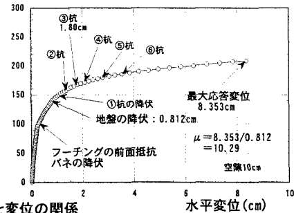
図6. 荷重と変位の関係
