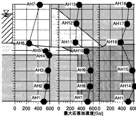
図-4 水平応答加速度の最大値分布
