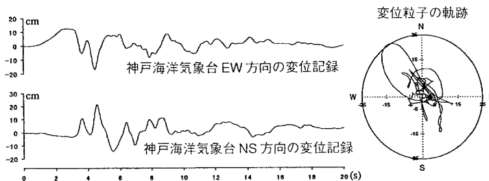
図2 入力地震動
