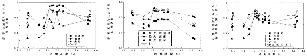
図-2 最大応答との相関係数と建物固有周期との関係図
