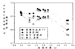
図-4 累積 \bar{a}_r による相関係数と建物固有周期との関係図
