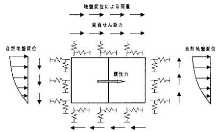
図-2 応答変位法概略図
