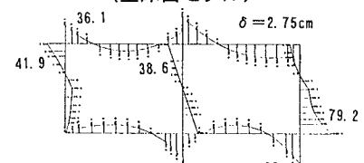
図-9 応答変位法 (FEM応答変位法)
