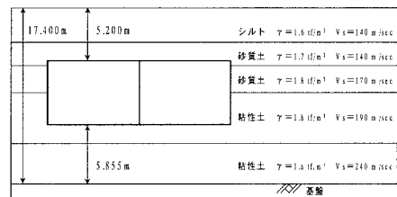
図-3 地盤モデル
