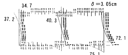
図-6 強制変形法 (動的解析)
