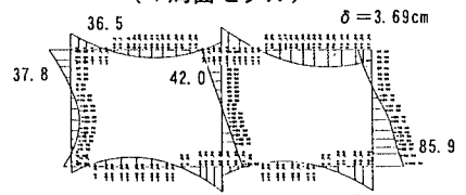
図-8 応答変位法 (上床面モデル)
