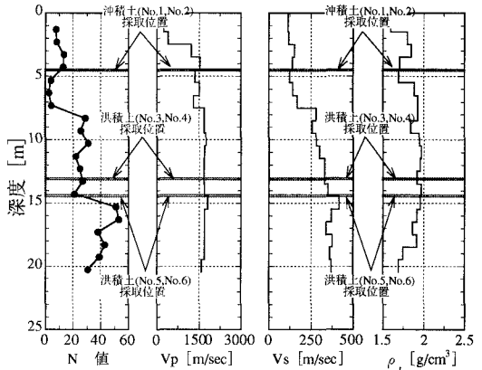
図-1 原位置試験結果
