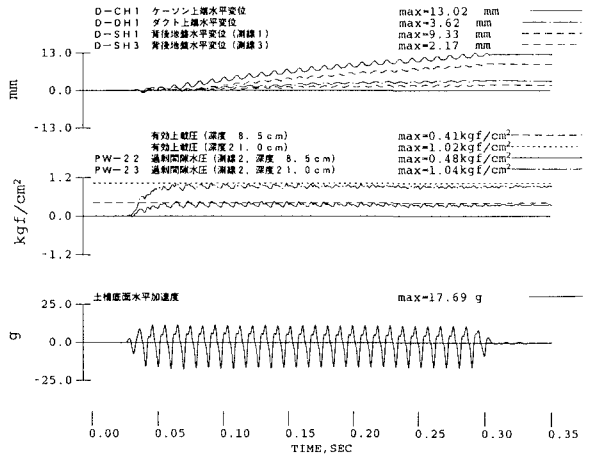
図-2 変位及び過剰間隙水圧波形
