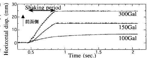
図-6 模型壁水平変位の経時変化
