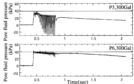
図-4 過剰間隙水圧の経時変化（300Gal）
