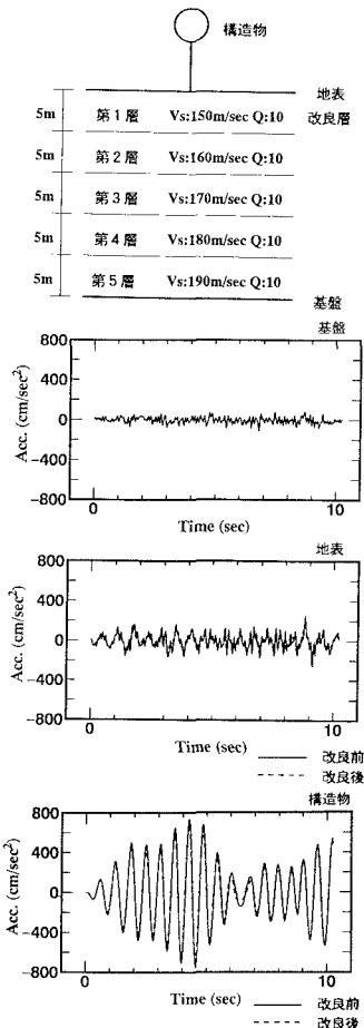
図-1 モデル地盤と応答加速度
