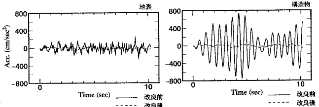
図-3 第3層を改良したときの地表面と構造物の加速度時刻歴
