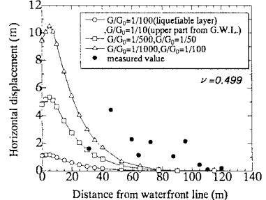
図4 地表面の水平変位量分布(昭和大橋)
