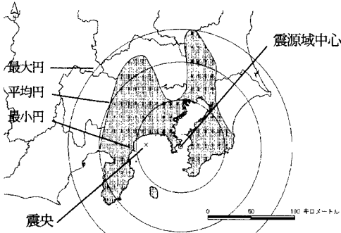
図2 関東地震（1923年、M7.9）の震度VIIに対する最大円、平均円、最小円
