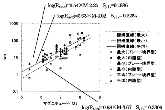
図3 最大距離、平均距離、最小距離とマグニチュードの関係（上：震度V、下：震度VI）
