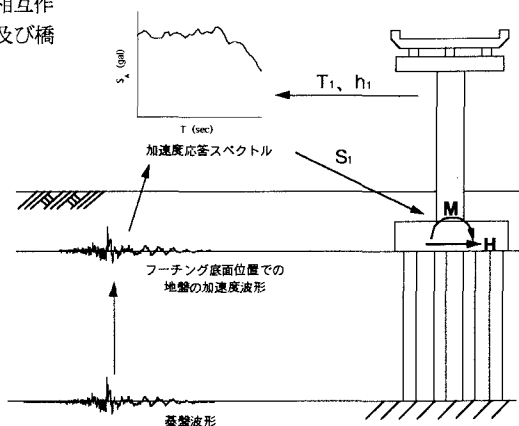
図-2 動的解析と比較をするための設計水平震度の考え方
