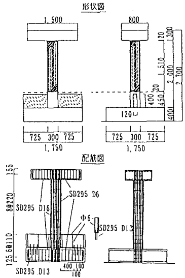
図—3 布基礎の有る試験体（CASE 3）
