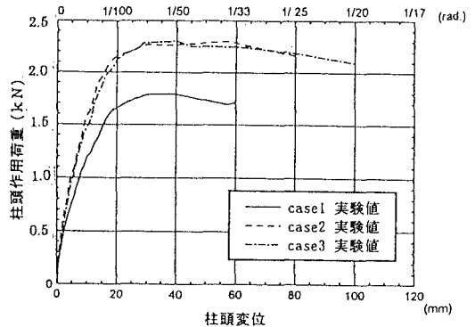
図—4 荷重・変位図
