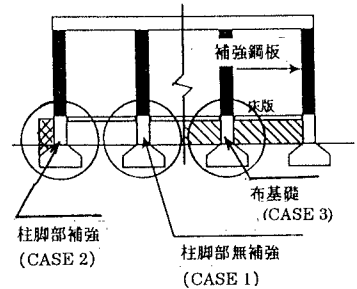
図-1 駅部高架橋補強法図 形状図
