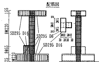
図-2 柱脚部補強試験体(CASE 2)
