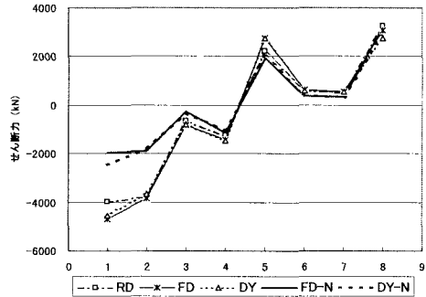
図3 断面力の比較
