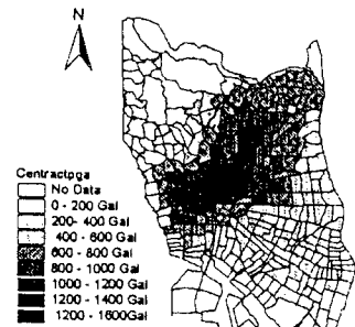
図6 地震動応答解析(FDEL 5) による地表面応答加速度分布
