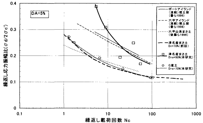
図-2 液状化強度曲線の比較
