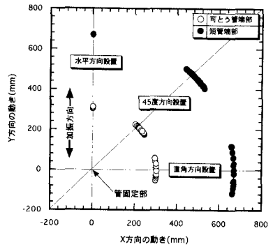
図-4(a) 管の水平面上の動き
