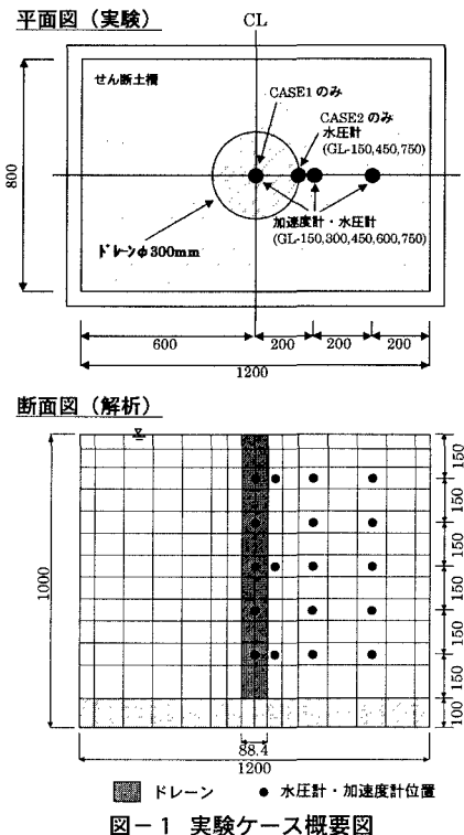
図-1 実験ケース概要図
