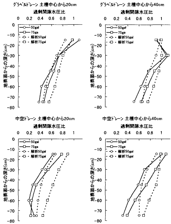
図-2 最大過剰間隙水圧比の深度分布
