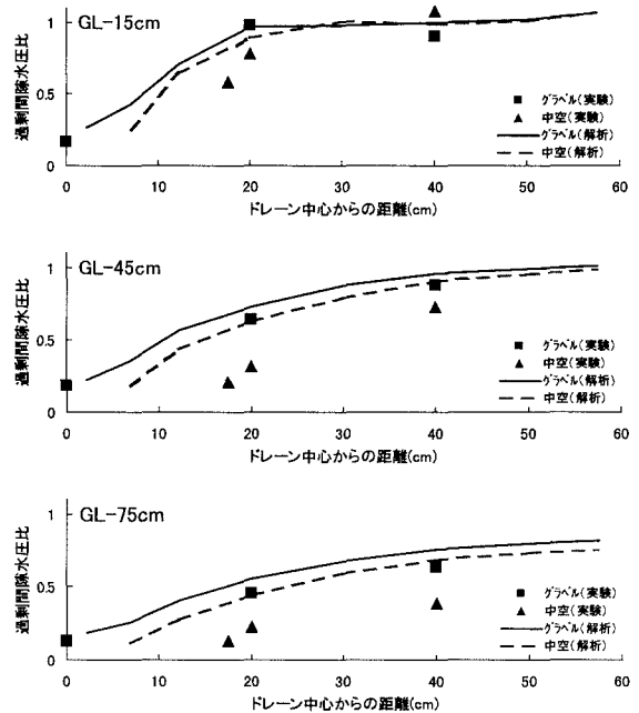
図-3 最大過剰間隙水圧比の水平方向分布図（75gal加振時）
