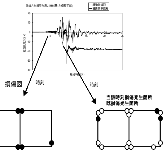
図-2 相互作用力時刻歴波形 (粘性土地盤、左側壁下部)
