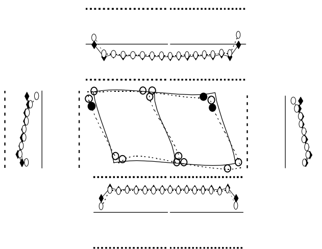
図-6 接線方向相互作用力(粘性土地盤)
