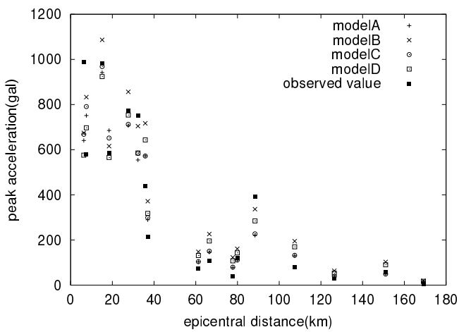
図 3: 台湾・集集地震の最大加速度と震央距離の関係
